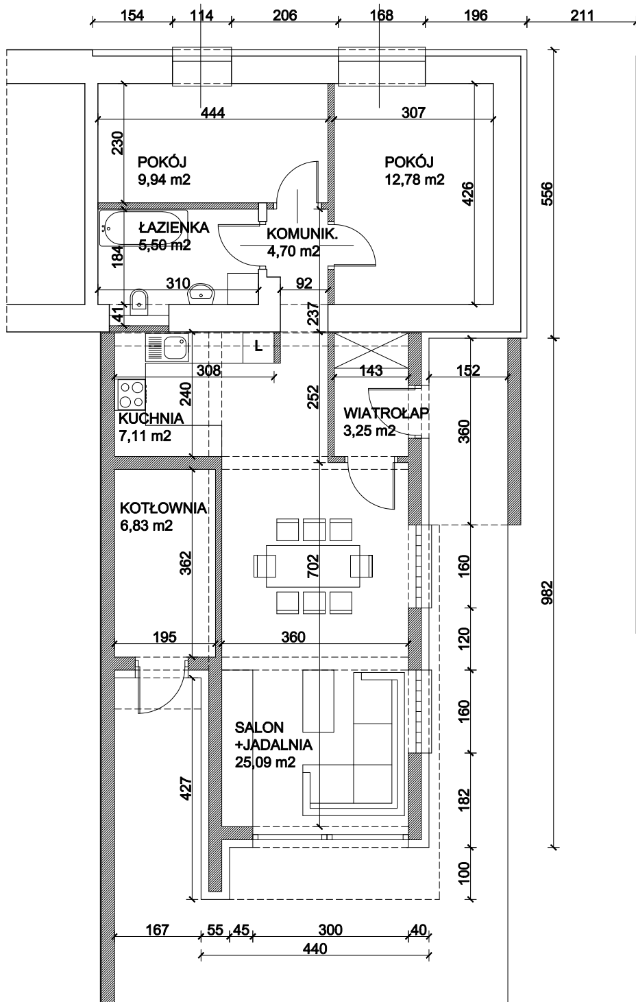
KONCEPCJA NR 2 POW. UŻYT. : 75,20 m 2
