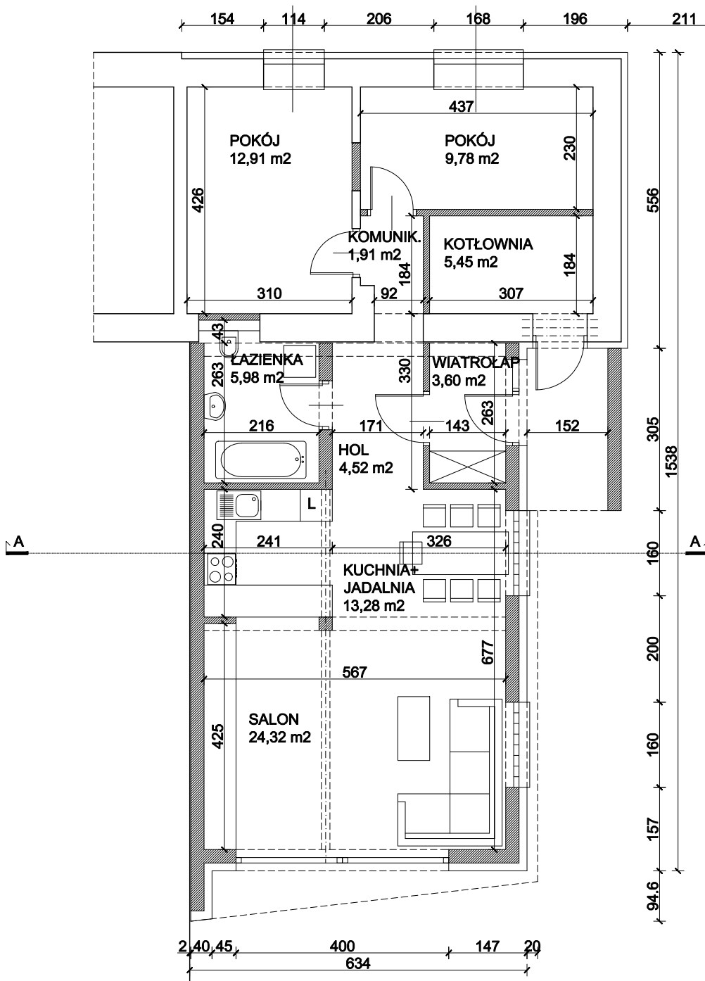
KONCEPCJA NR 1 POW. UŻYT. : 81,75 m 2
